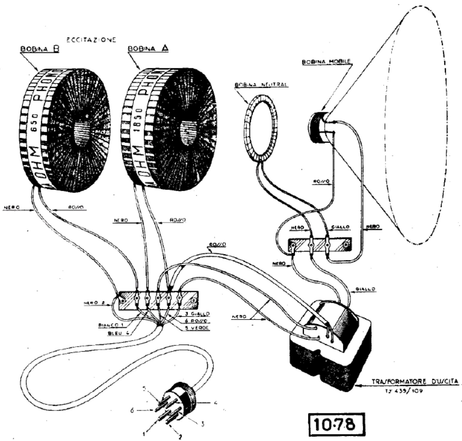
Gli elementi della parte tonica del mod. « 880 ». Piano dei componenti l'altoparlante elettrodinamico.
